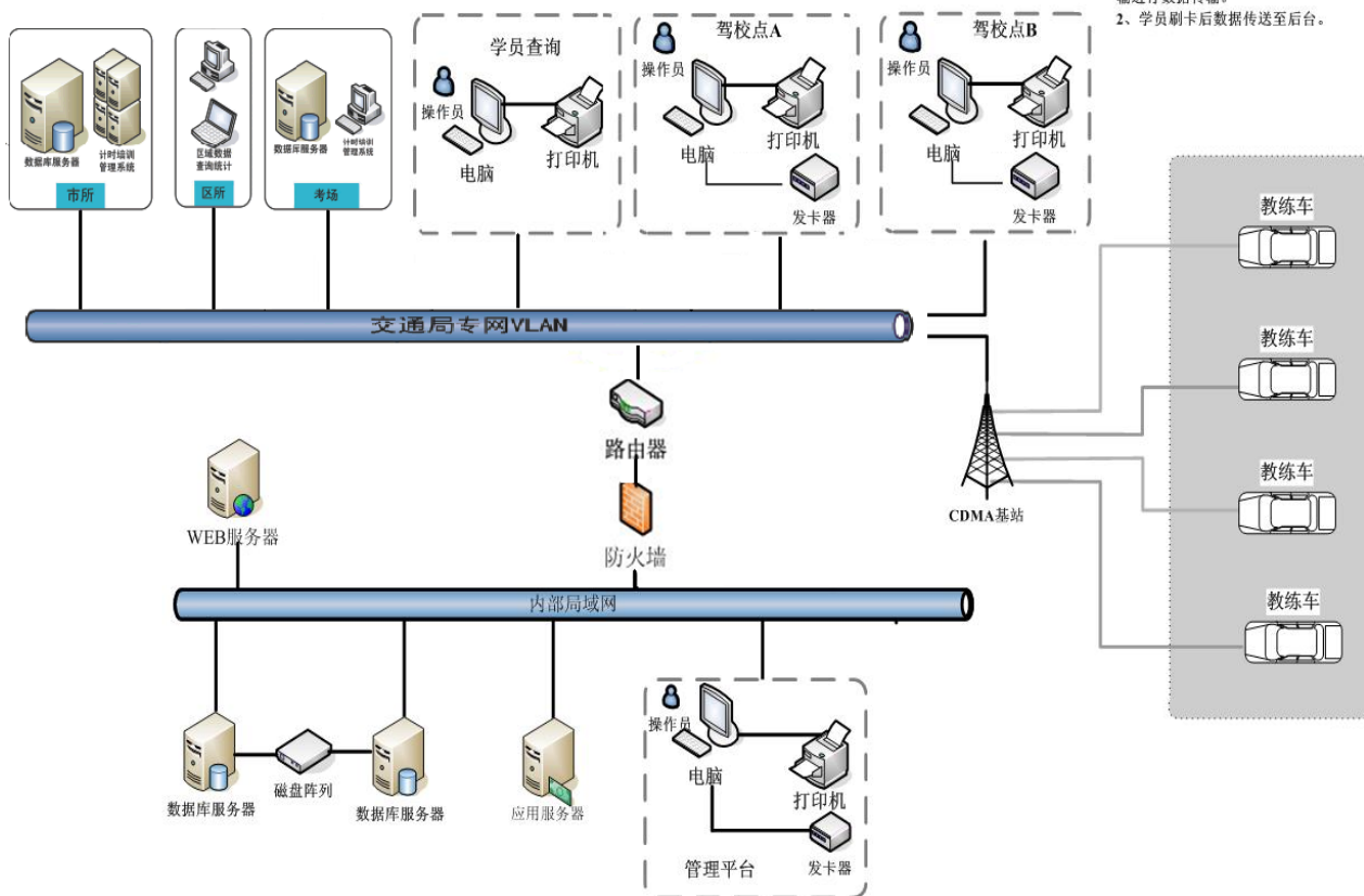
2G/3G无线驾校一卡通管理系统拓扑图
